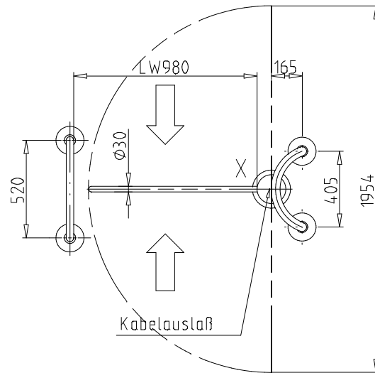
Detail X: Drehsternflansch M 1:5
