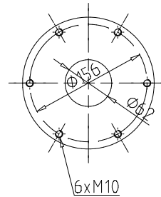
Detail X: Drehsternflansch M 1:5
